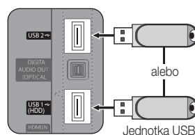
Zadný panel TV
