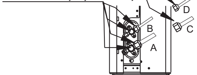
A: Zaporni ventil niskog tlaka B: Zaporni ventil visokog tlaka C & D: Matice unutarnjeg dijela
