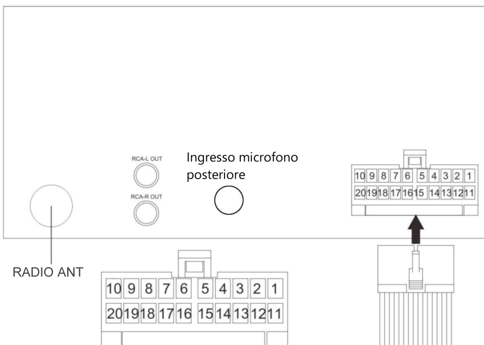
VISTA INSERIMENTO CAVO
