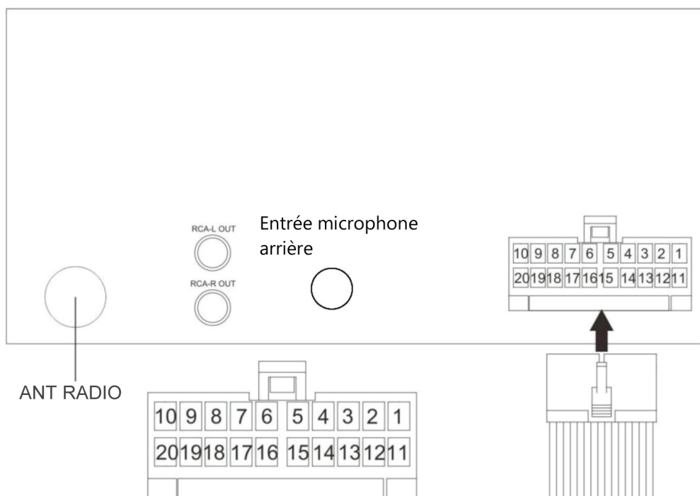
VUE D'INSERTION DU CÂBLE
